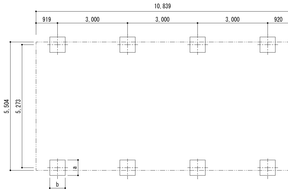
■基礎配置図
